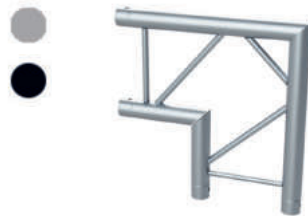
Esquina truss paralelo. 2 vías. 90°. 300mm. Tubo principal: 50x2mm. Tubo secundario: 16x2mm. Plateado o negro. SERIE F
