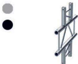
Esquina truss paralelo en cruz. 4 vías. 300mm. Tubo principal: 50x2mm. Tubo secundario: 16x2mm. Plata o negro. SERIE F
