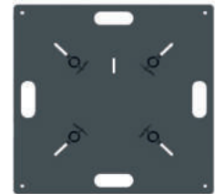
Base cuadrada para truss cuadrado, triangular y paralelo, truss desde 29mm hasta 40mm, Serie E
