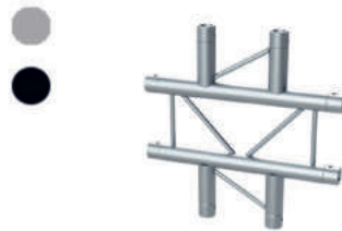
Esquina truss paralelo en cruz. 4 vías. 250mm. Tubo princ: 50x2mm. Tubo sec: 13x1,5mm. Plata o negro. SERIE F
